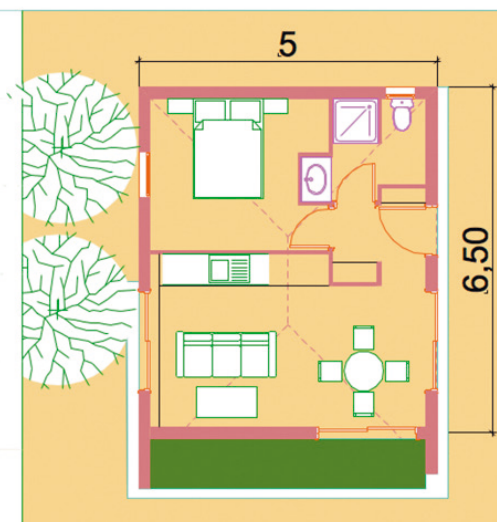
Maisonnette 7 x 7 m et 5 x 6,50 m en terre, paille + toit panneaux solaires + potager + terrasses
